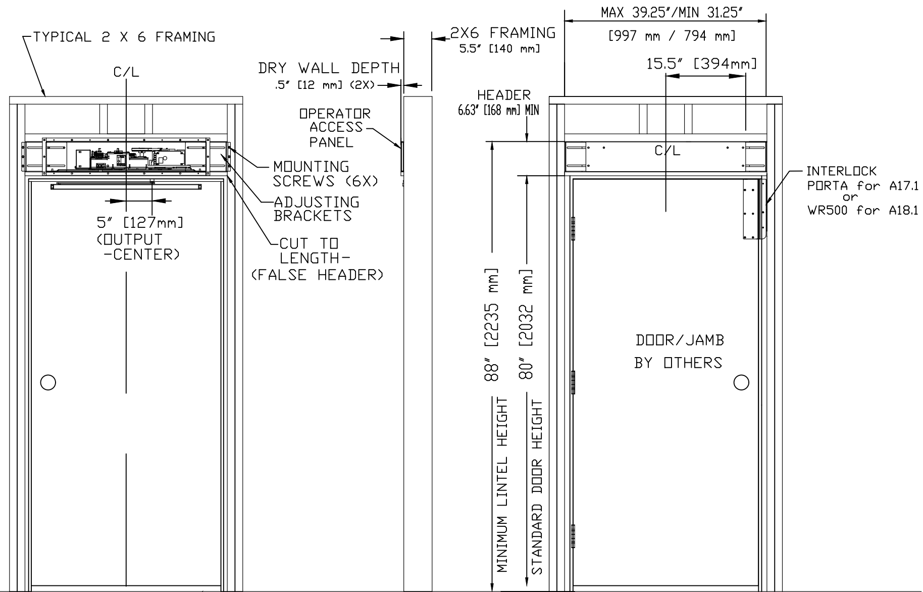
FRONT VIEW (LANDING)
